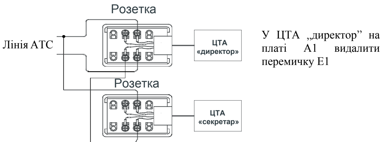
Рисунок 2 – Підключення до абонентської лінії двох телефонних апаратів за схемою «ДИРЕКТОР-СЕКРЕТАР»
