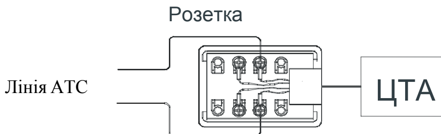
Рисунок 1 – Схема підключення телефонного апарата до абонентської лінії
